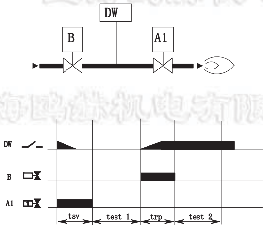
附图表，显示该装置的工作循环状态
